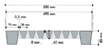
Caillebotis largeur 500 :
