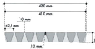
Caillebotis largeur 420 :
